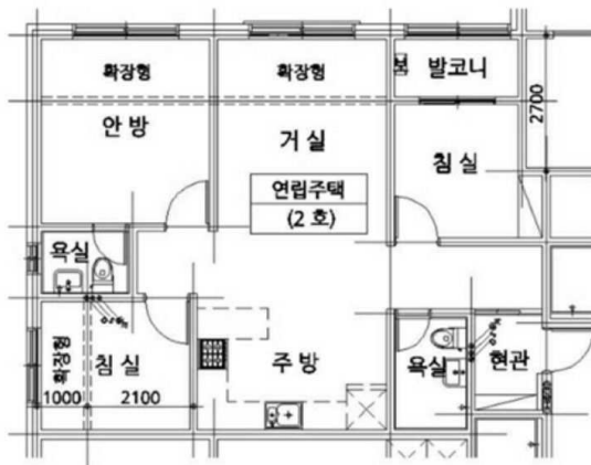
< 호별배치도 > 제5층 제502호
