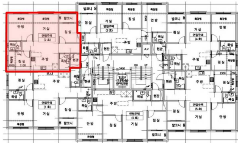
< 호별배치도 > 제5층 제502호
