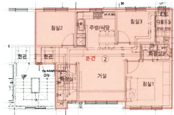
<내부구조도>
