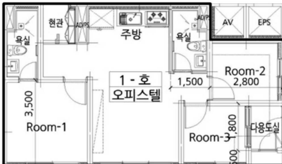
< 내부구조도 >
