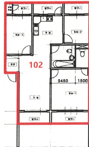
[내부구조도]
