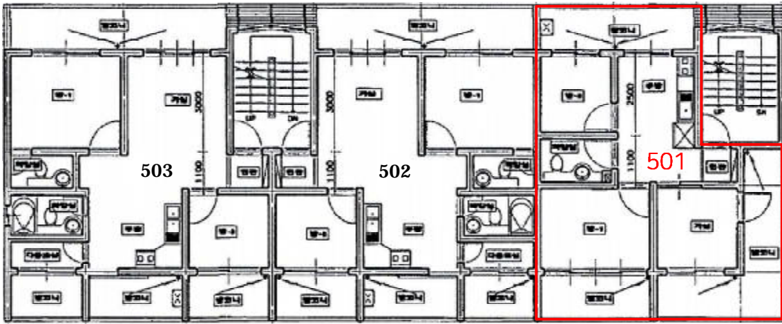
< 호별배치도 >
