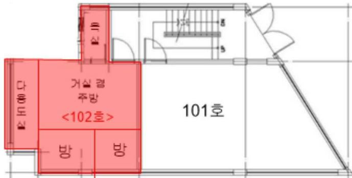
< 일련번호 5) 호별 배치도 >
