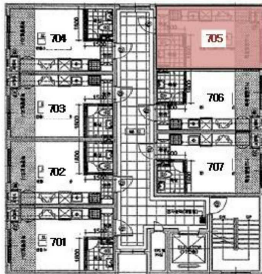
< 7층 호별배치도 >
