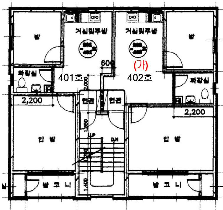
[호별배치도]
