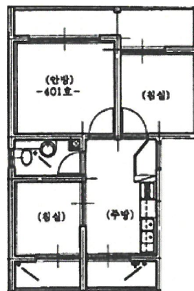
< 동부주택 제4층 제401호 내부구조도 >
