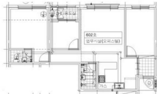
< 내 부 구 조 도 >
