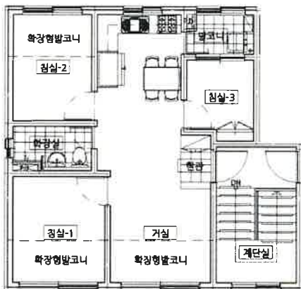
<제4층 제405호 내부구조도>
