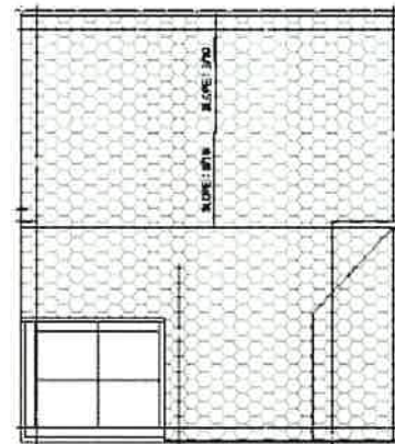
<지붕층 평면도>
