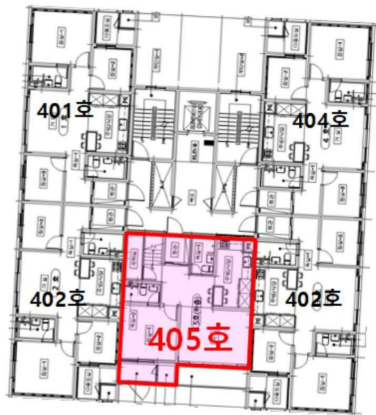
[호별배치도]
