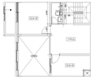
[5층 내부구조도]
