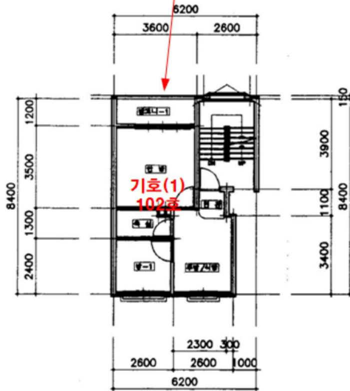
호별 배치 및 내부구조도
