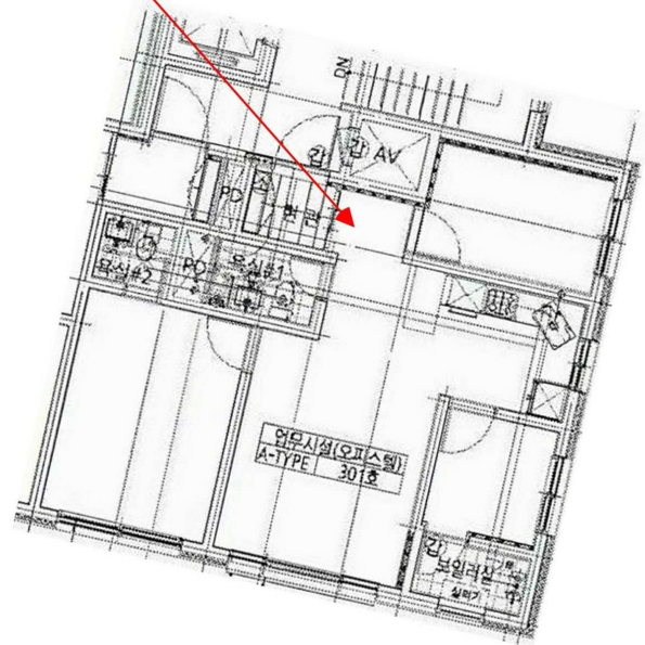
[제3층 제301호 내부구조도]
