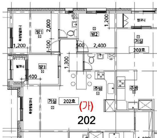
[내부구조도]
