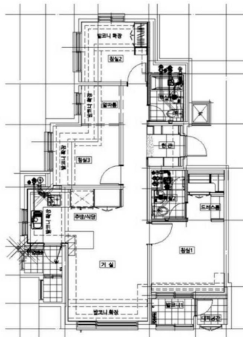
< 호별 배치도 > 제5층 제506호
