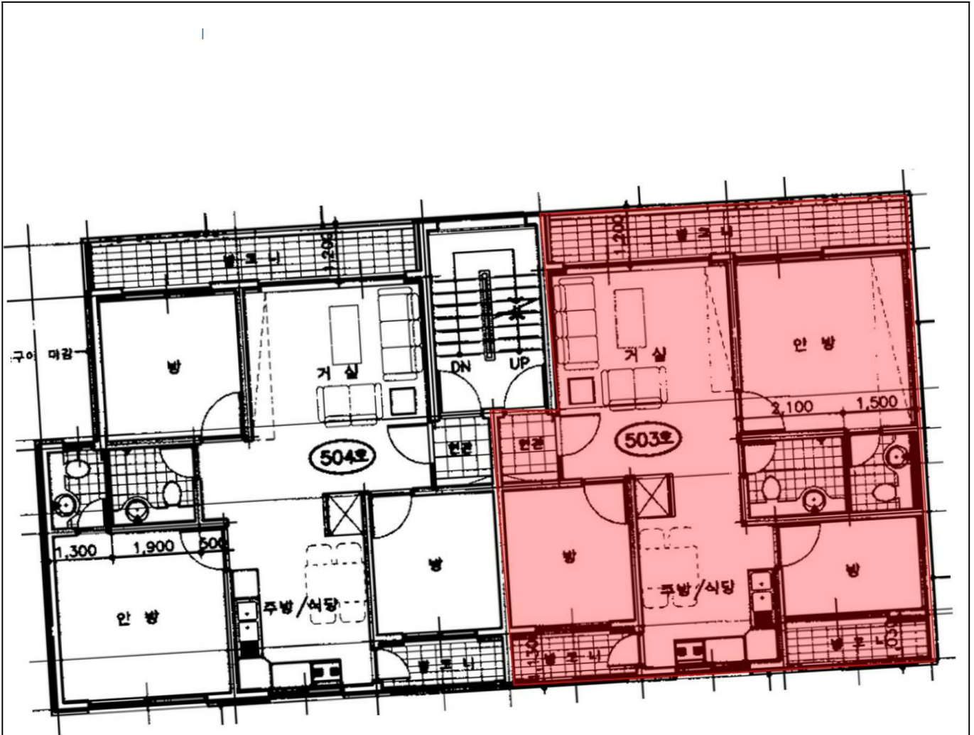
5층 503호 내부구조도
