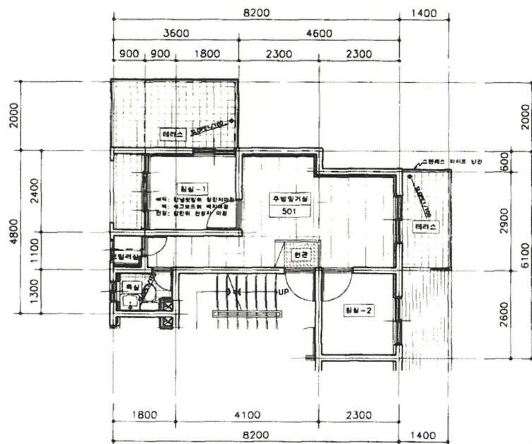
[ 경기도 부천시 소사구 심곡본동 742-8번지 제5층 제501호 내부구조도 ]
