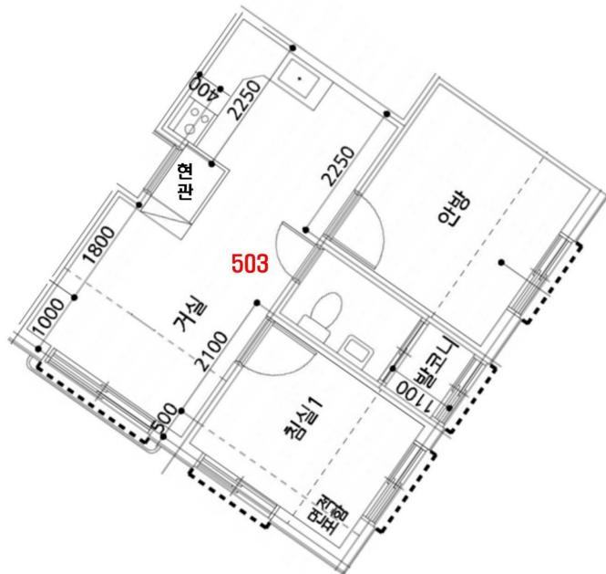
< 내부구조도 >
