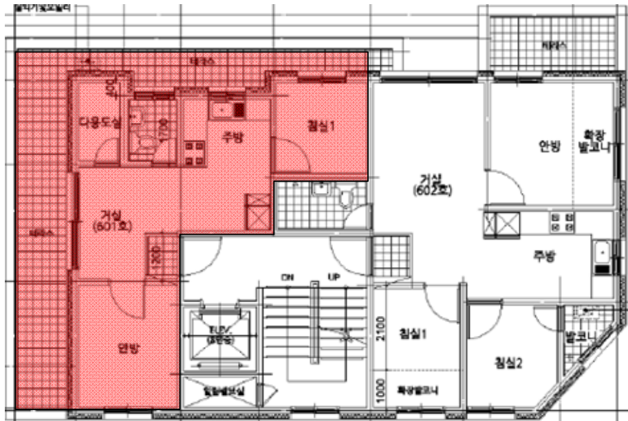
내부구조도 (601호)
