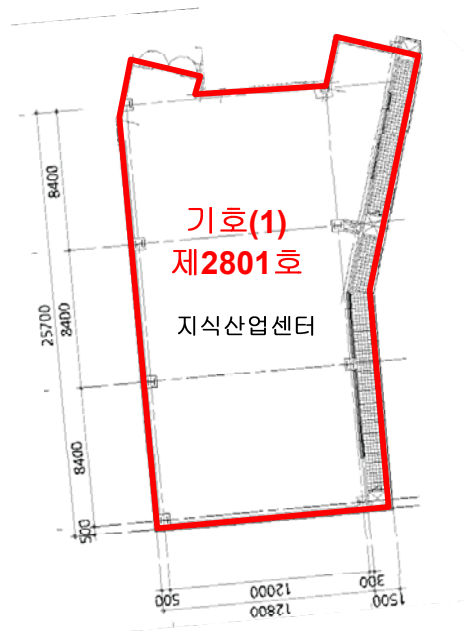
< 제2801호 내부구조도 >
