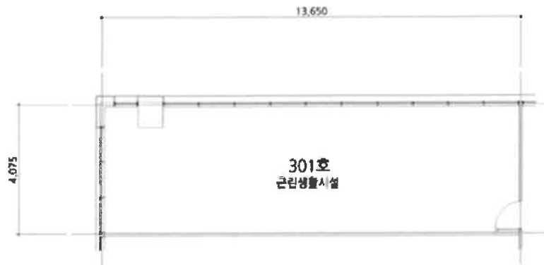
< 내부구조도 >
