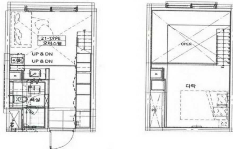
< 내부구조도 >
