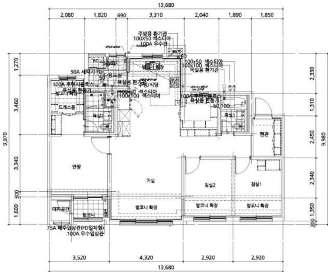
[ 서봉마을모아엘가 801동 4층 401호 평면도 ]
