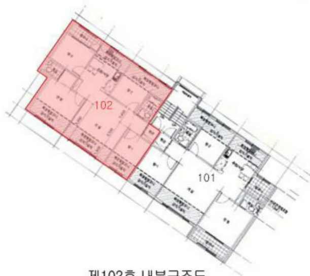
제102호 내부구조도
