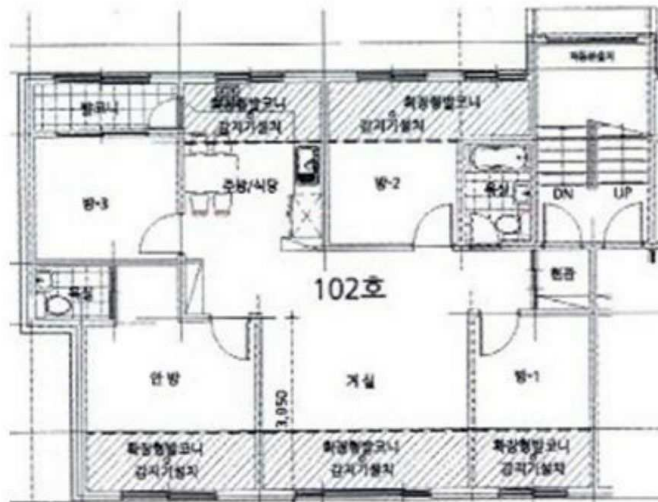
제102호 내부구조도
