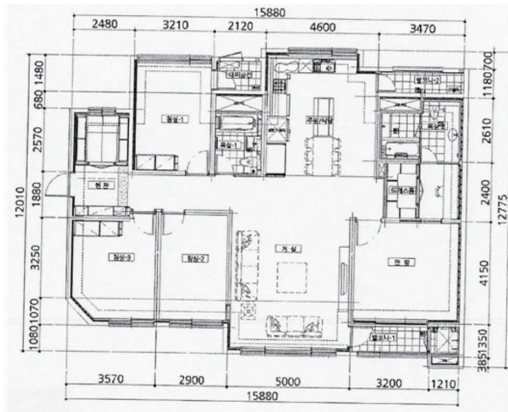
[내부구조도]
