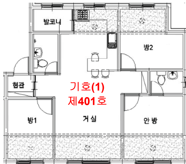
< 제401호 내부구조도 >
