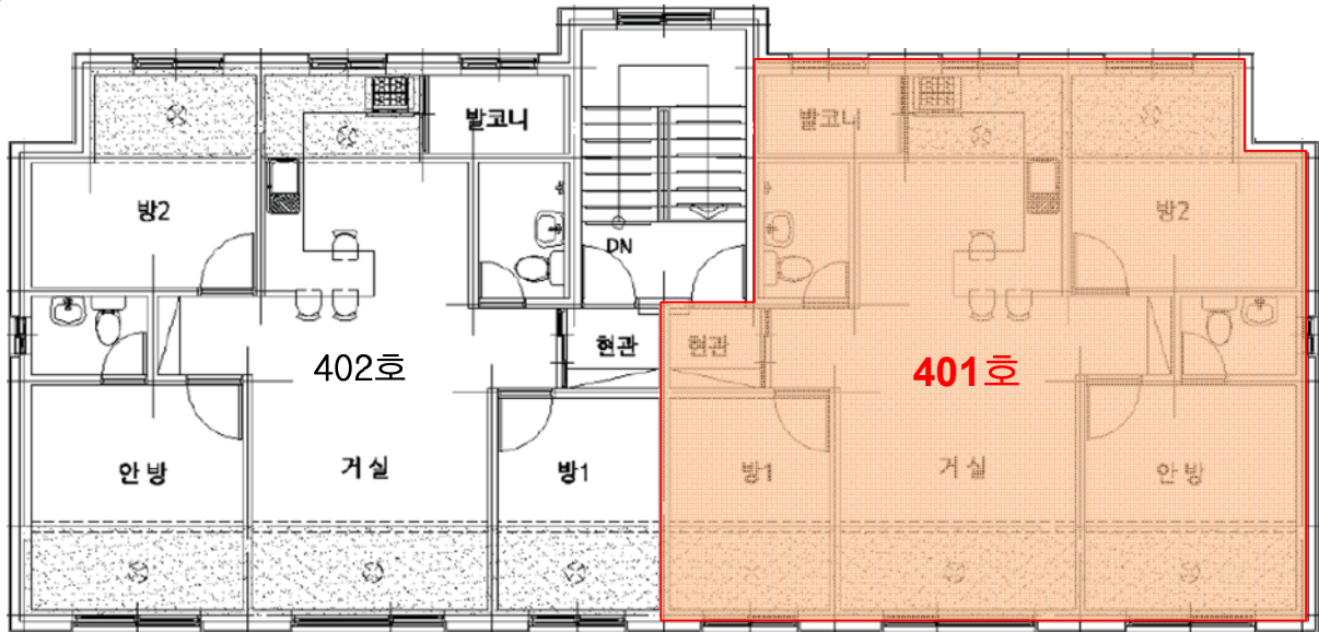
< 제5동 제4층 호별배치도 >
