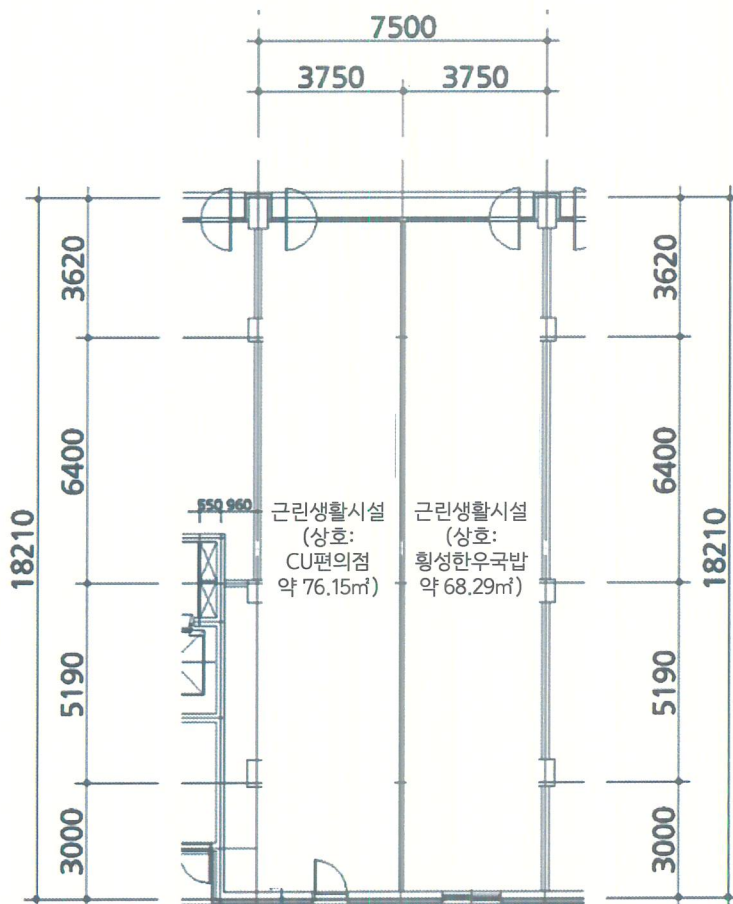
< 제상가103호 내부구조도 >
