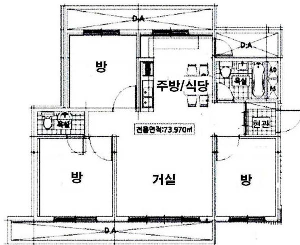
(비01호 내부구조도)
