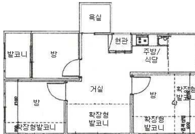
[ 내부구조도 ]
