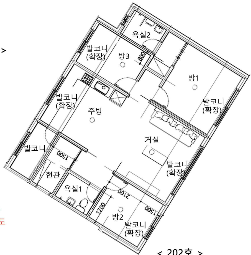
[ 내부 구조도 ]
