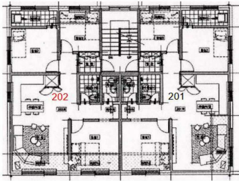
<2층 평면도>
