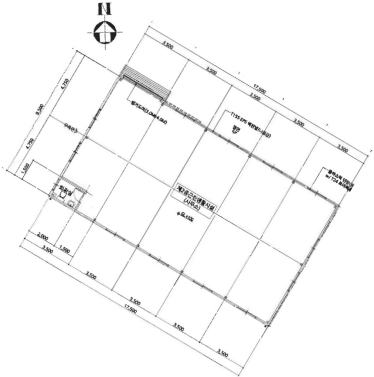
기호(4) 평면도
