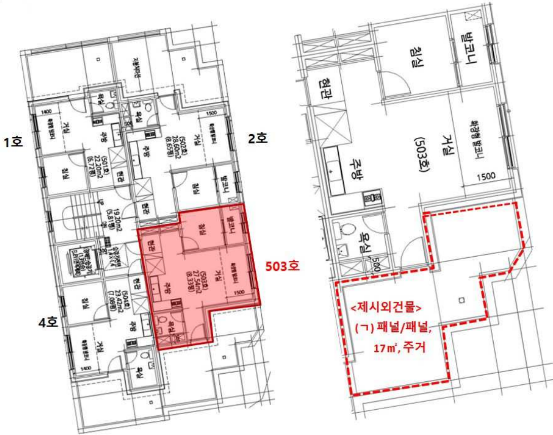
<제5층 호별배치도>
