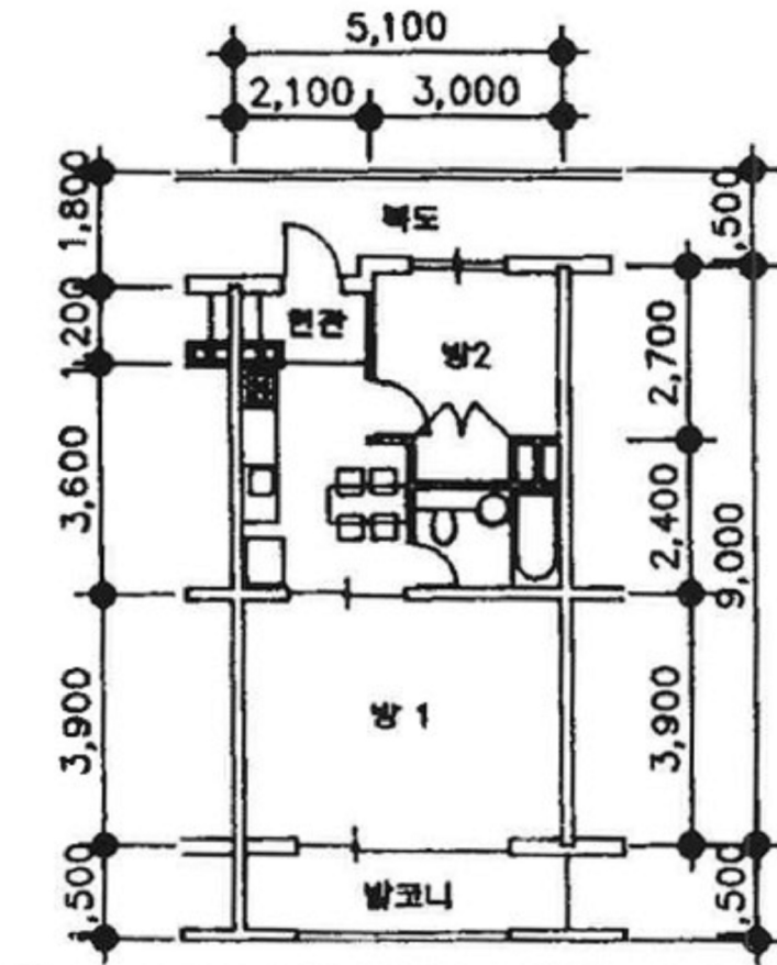
[ 내부구조도 ]
